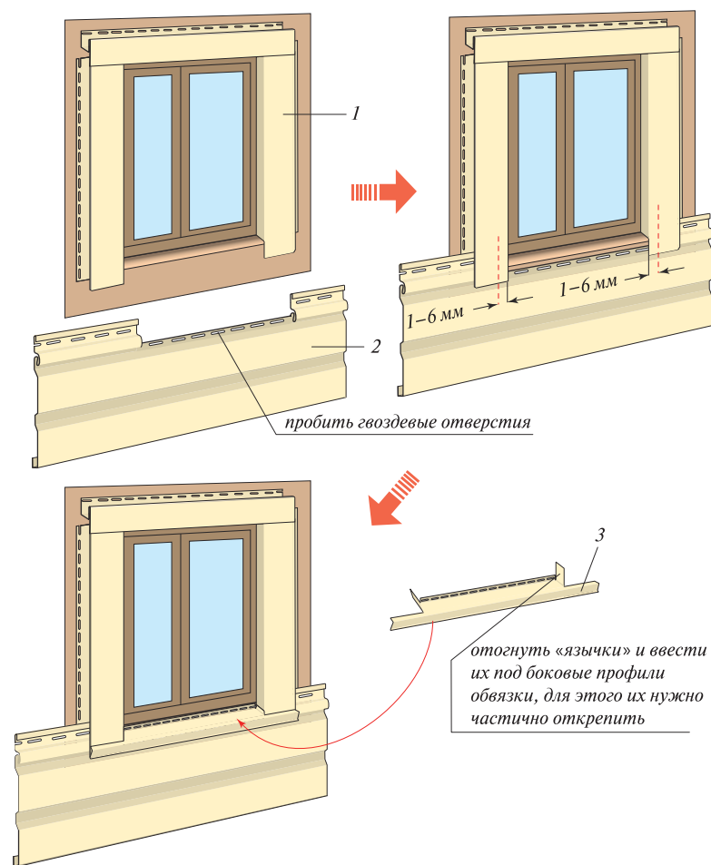
Рис. 36. Установка сайдинга вокруг проемов на обычных крепежах (гвоздях или саморезах): 1 – обвязка окна околооконным профилем; 2 – рядовая сайдинговая панель; 3 – отлив Döcke
