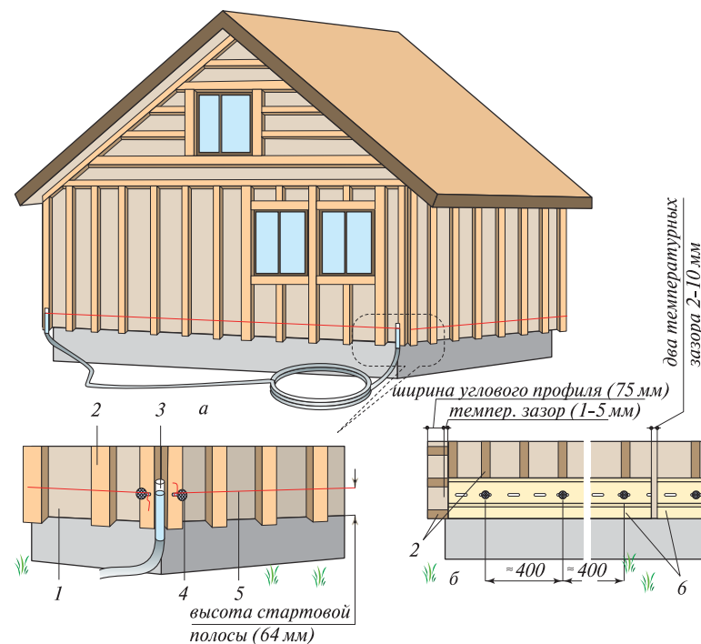
Рис. 16. Монтаж стартового профиля (размеры в мм): а — отбивка горизонта; б — установка стартовых полос; 1 — стена; 2 — обрешетка; 3 — водяной уровень; 4 — гвоздь; 5 — шнурок; б — стартовая полоса
