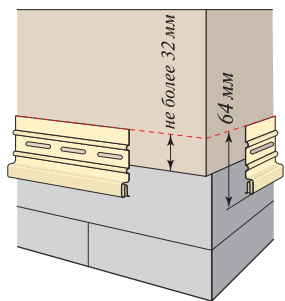
Рис. 17. Нанесение обшивки на цоколь
