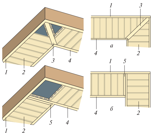
Рис. 53. Соединение софмитных подшивок на углах: а — на косой угол; б — на прямой угол; 1 — карнизный принимающий профиль; 2 — софмит; 3 — Н-профиль или два J-профиля; 4 — пристенный принимающий профиль; 5 — J-профиль
