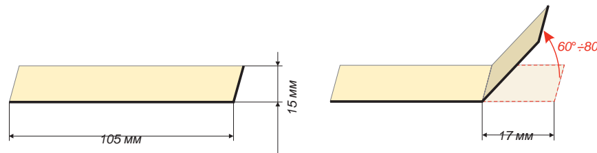
Рис. 25. Изготовление скобы и вставки
