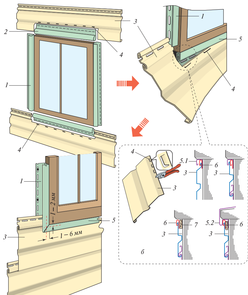
Рис. 35. Установка сайдинга вокруг проемов на «зацепах»: а – общая схема монтажа; б – варианты узлов нижней (и верхней) обвязки; 1 – боковой профиль обвязки проема (J-профиль, наличник или околооконный профиль); 2 – верхний профиль обвязки; 3 – рядовая сайдинговая панель; 4 – зацеты; 5 – нижний профиль обвязки (5.1 – J-профиль или наличник, 5.2 – околооконный профиль); 6 – финишный профиль; 7 – выравнивающая высота деревянная рейка
