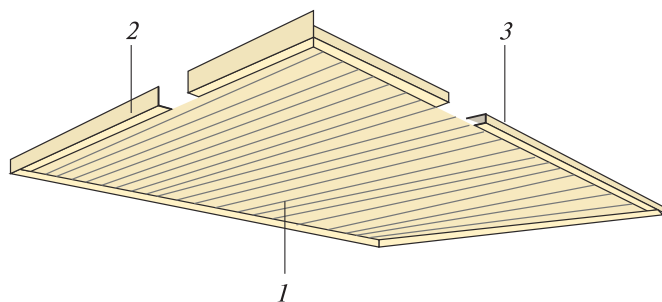
Рис. 54. Пример устройства софмита над открытой верандой: 1 — софмит; 2 — фаска; 3 — J-профиль или молдинг
