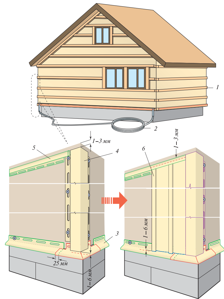
Рис. 45. Схема монтажа вертикального сайдинга: 1 — горизонтальная обрешетка; 2 — водяной уровень; 3 — отлив Дёске; 4 — угловой профиль; 5 — J-профиль; 6 — вертикальный сайдинг (неперфорированный соффит)
